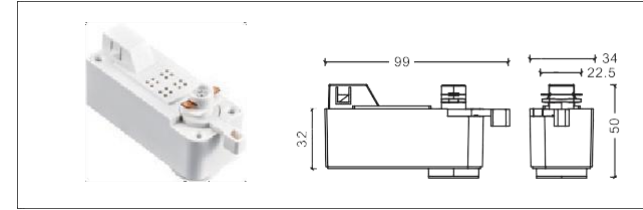
NO: AE-211 2 線小軌道盒
