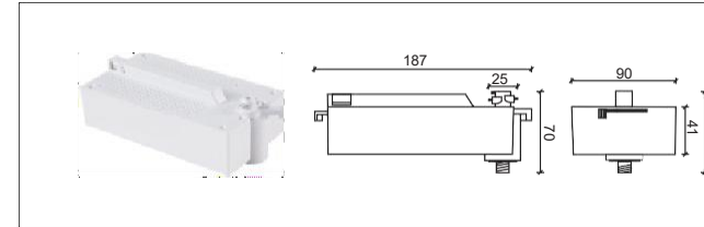
NO: AE-212 2 線一體電氣箱
