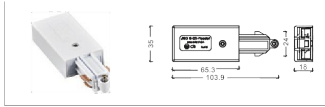
NO: AE B-02-feeder 假3線電源頭
