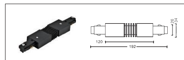
3線短軟接頭 Connector
