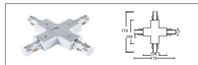
3線A十字接頭 X-connector
