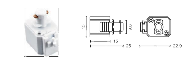
NO: 2 線迷你軌道頭
