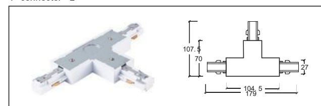
3線A T接頭-左 T-connector - L
