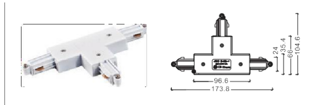
NO: AE B-02-T 假3線T接 高壓
