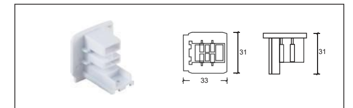
H-04 尾蓋 End cap
