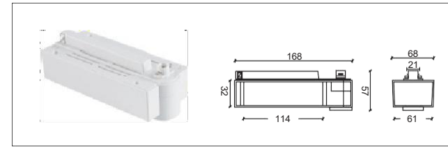
NO: AE-218 2 線簡易電氣箱
