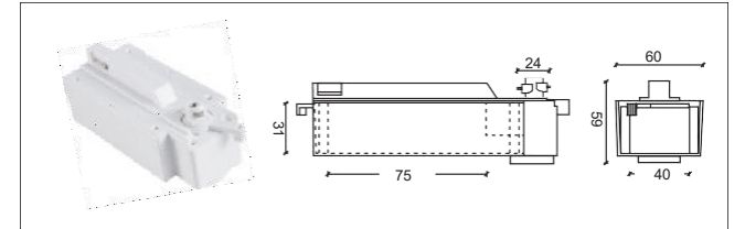
NO: AE-219 2 線短電氣箱
