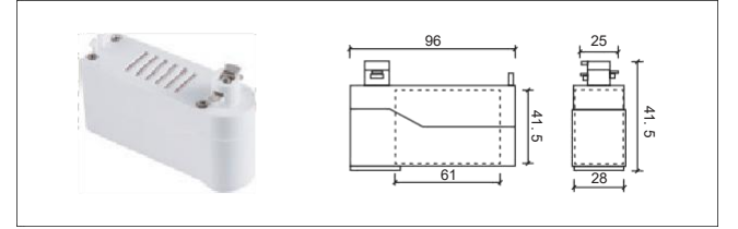
NO: AE-313 3 線簡體電氣箱
