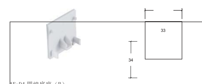
AE-D4 四線底座 (B)
