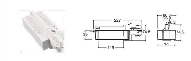
NO: AE-406 4 線大電氣箱
