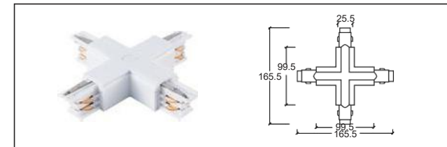
H-04 十字接頭 X-connector
