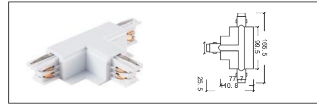
H-05 T接頭-左 T-Connector - L
