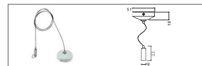
3線掛件吊裝線 Fitting
