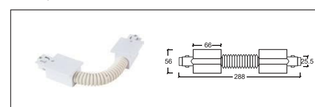
H-03 多角度接頭(軟接) Flexible Connector
