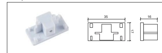
3線A尾蓋 End cap
