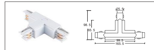
H-04 T接頭-左 T-connector - L
