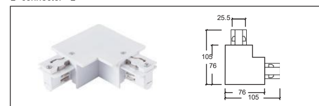
H-03 L 型接頭-左 L-connector - L
