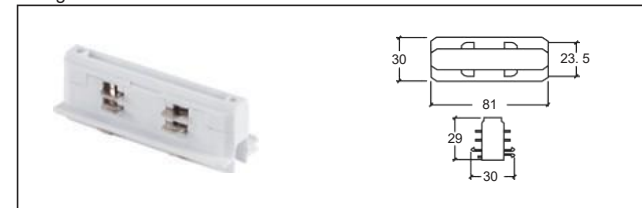
H-02 迷你型直線接頭 Straight connector MINI
