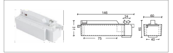
NO: AE-306 3 線短電氣箱
