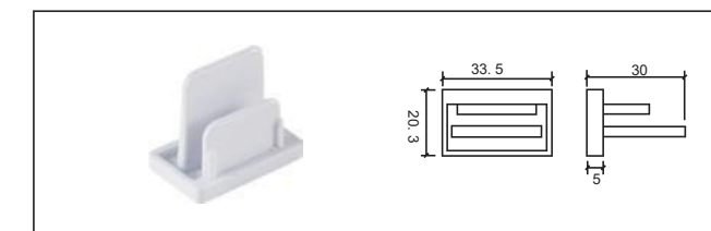
2線L 型接頭
