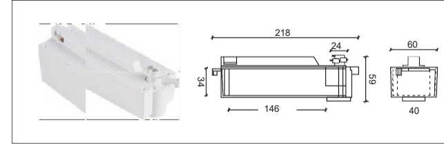
NO: AE-311 3 線長電氣箱
