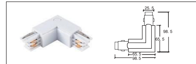
H-04 L 型接頭-左 L-connector - L
