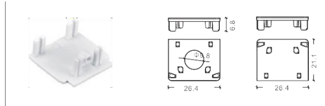
NO: 2 線迷你軌道條尾蓋
