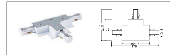
3線A 嵌入式T接頭-右 T-connector - R
