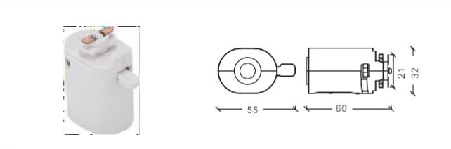
NO: K206 韓國 2 線軌道頭
