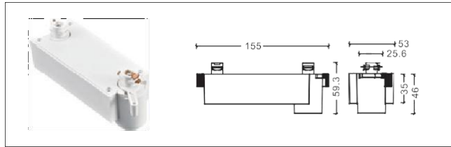
NO: AE-328 3 線雙柄電器盒
