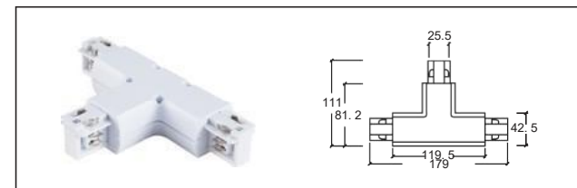
H-01 T接頭-左 T-connector - L
