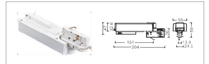
NO: AE-469 配 AE-412
