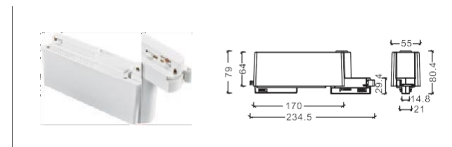
NO: AE-266 配 AE-209 軌道條
