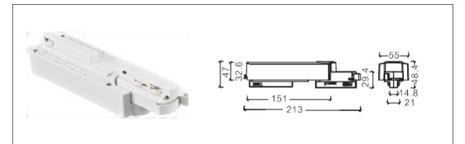
NO: AE-269 配 AE-209 軌道條
