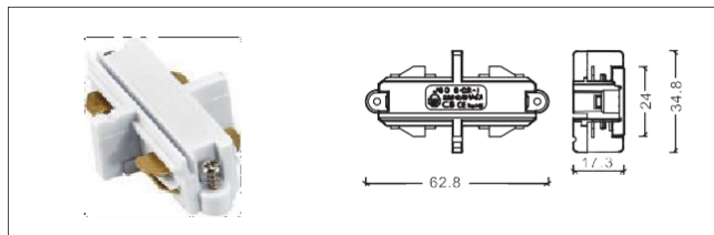
NO: AE B-02-I-NIMI 假3線內接
