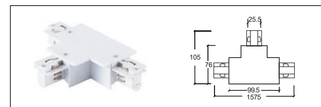
H-03 T接頭-左 T-connector - L
