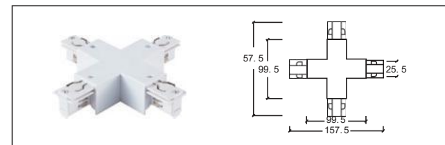
H-02 十字接頭 X-connector
