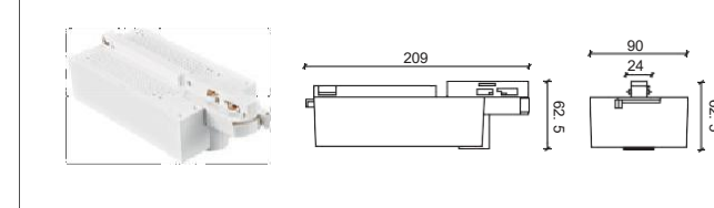
NO: AE-304 3 線大電氣箱
