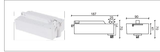
NO: AE-305 3 線一體電氣箱
