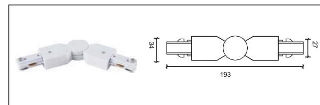
任意角度接頭 Flexible Connector
