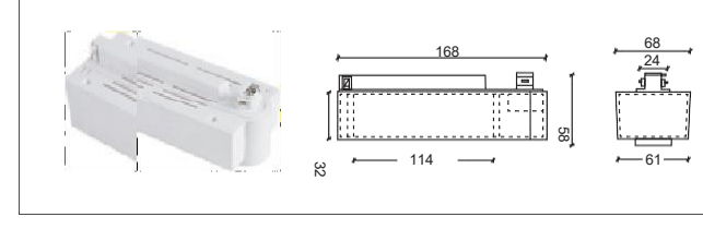
NO: AE-314 3 線簡易電氣箱
