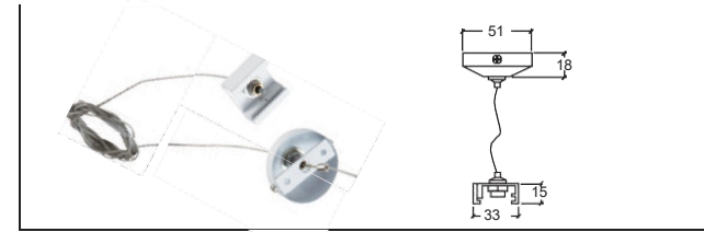
H-04 線軌道吊裝線 Fitting
