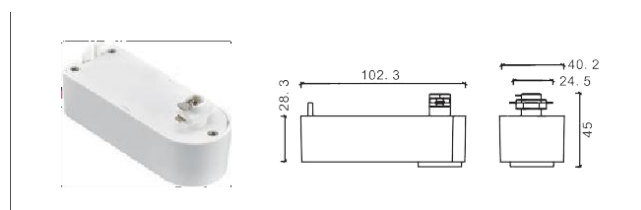
NO: AE-300 3 線迷你電器盒
