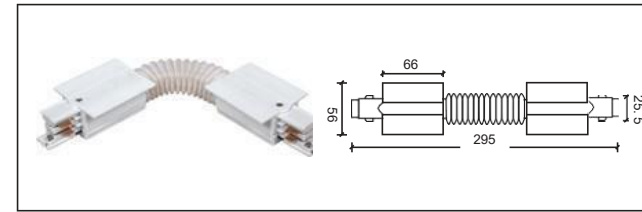
H-05 多角度接頭(軟接) Flexible Connector
