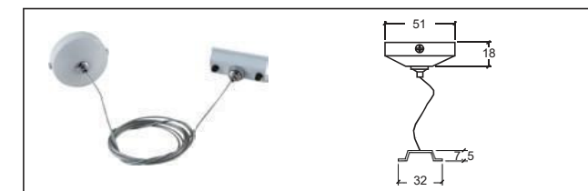
H-02 四線吊裝線 Fitting
