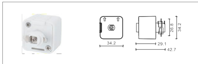
NO: AE-302 (S) 3 線小方盒軌道頭
