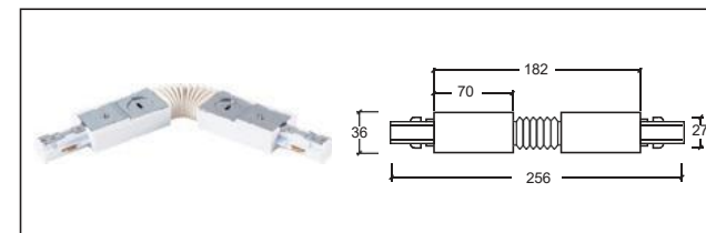
3線A多角度接頭(軟接) Flexible Connector
