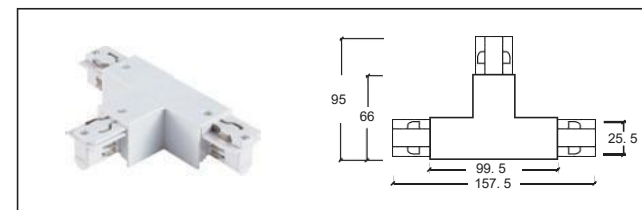
H-02 T接頭-左 T-connector - L
