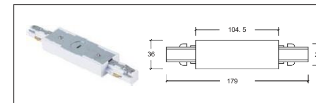
3線A直線接頭 Straight connector
