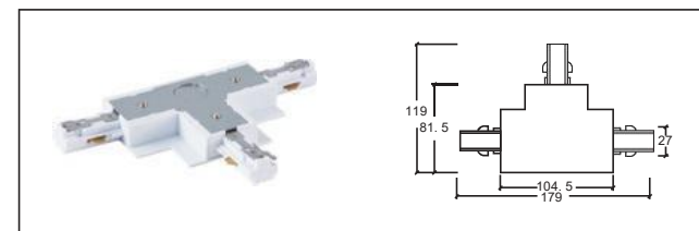
3線A 嵌入式T接頭-左 T-connector - L
